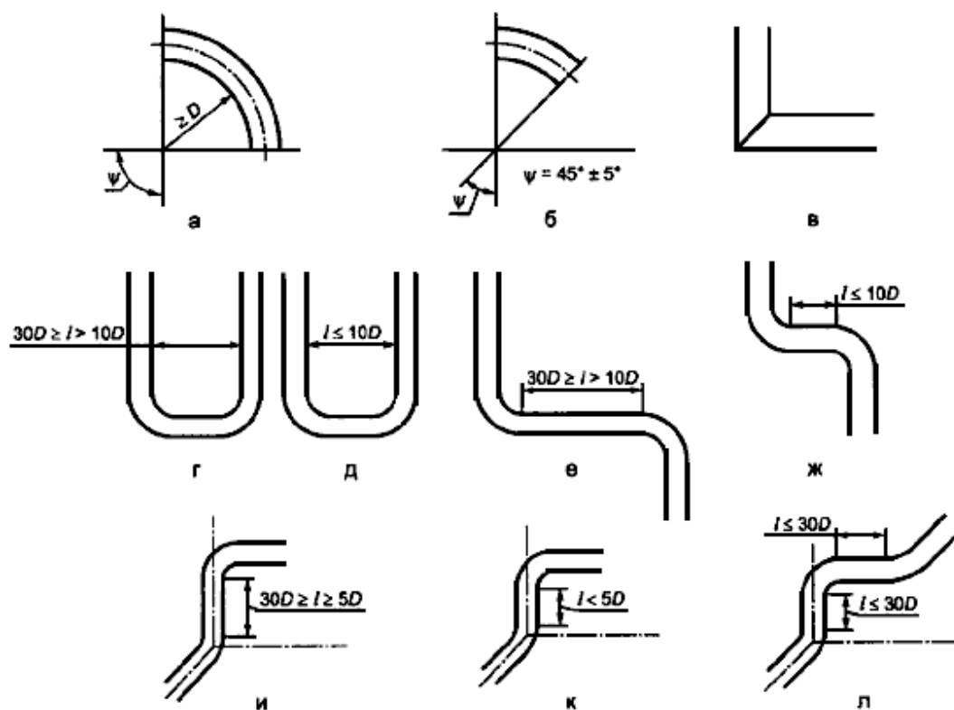
Рисунок А.1 - Колено и группы колен
