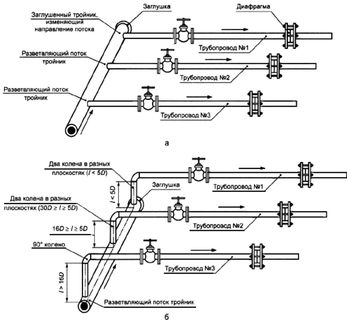
Рисунок 6 - Схема коллектора
