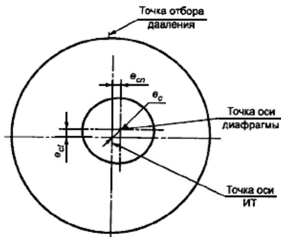
Рисунок 10 - Параметры эксцентриситета установки диафрагмы
